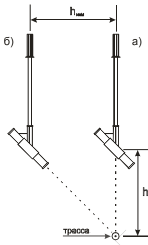
Рисунок 8. Определение глубины залегания трассы антенной 45°.
