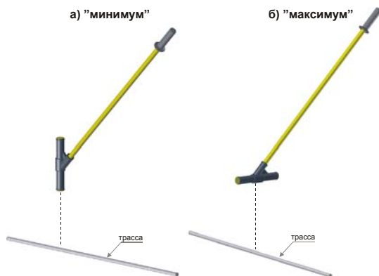
Рис 5. Положение антенны 45^\circ над трассой при поиске по «минимуму»- а) и по «максимуму» - б).
