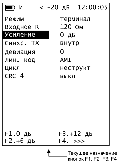
Рисунок 9-1. Меню настройки линейного интерфейса
