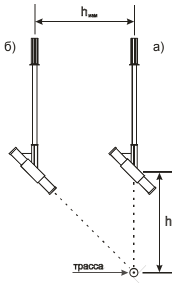
Рисунок 6. Определение глубины залегания трассы методом 45°.
