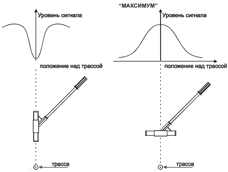
Рис. 5. Зависимость уровня сигнала от положения антенны над трассой и режима поиска.
