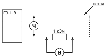
Рисунок 9.1. Схема для проведения проверки приемника.
