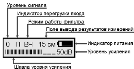
Рисунок 7.1. Жидкокристаллический дисплей.
