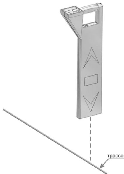
Рисунок 7.2. Рабочее положение приемника над трассой.
