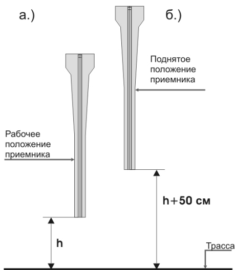
Рисунок 9.3. Положение приемника при настройке глубины залегания трассы.
