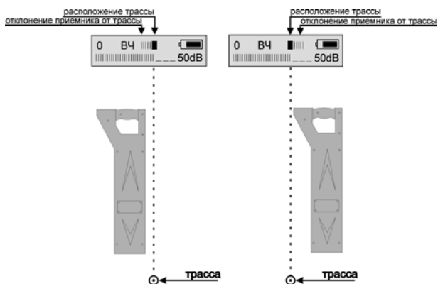
Рисунок 7.4. Положение приемника над трассой в режиме «MAX+» или «MIN»
