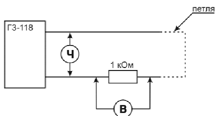
Рисунок 9.1. Схема для проведения проверки приемника.
